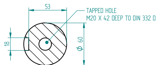
Przekrój A-A 1:2
